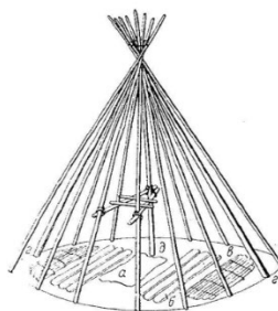
Устройство чума: а – очажный лист железа; б – доски пола; в – спальные циновки; г – два опорных шеста; д – очажный шест симзы.
