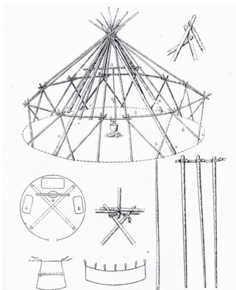
Рис. 1. Цилиндро-коническая юрта чорама-дю: остов жилища, способы скрепления верхушек основных жердей, план жилища, части остова, дверь, нижняя покрышка
